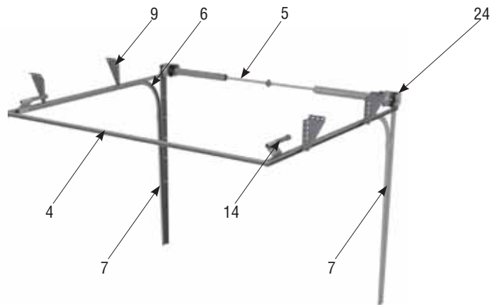
Система направляющих и торсионный механизм
